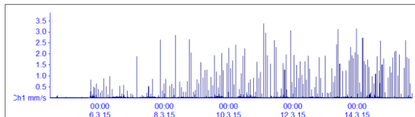
Erschütterungsmessung mit MR2002
